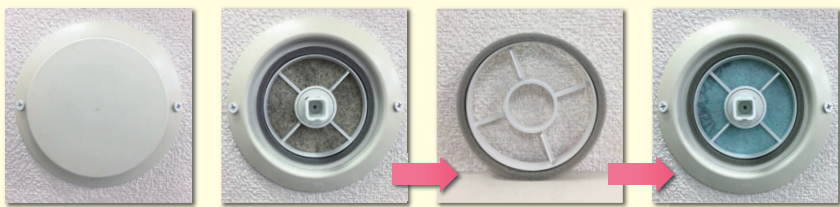
給気口(各部屋) カバーを外します 専用枠 フィルター取付後 「専用枠」がある場合は、再利用します。
